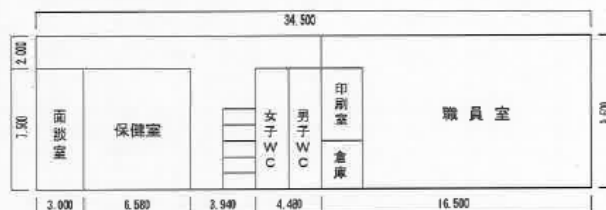
27 新館1階
