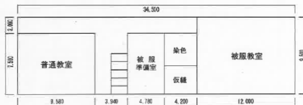
27 新館3階
